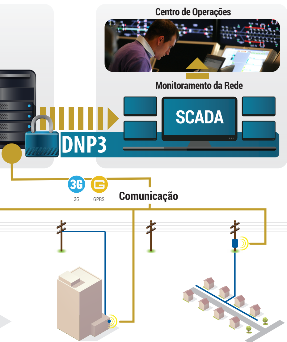
Ilustração do funcionamento do Módulo Front-end DNP3 com os módulos de comunicação CAS.
