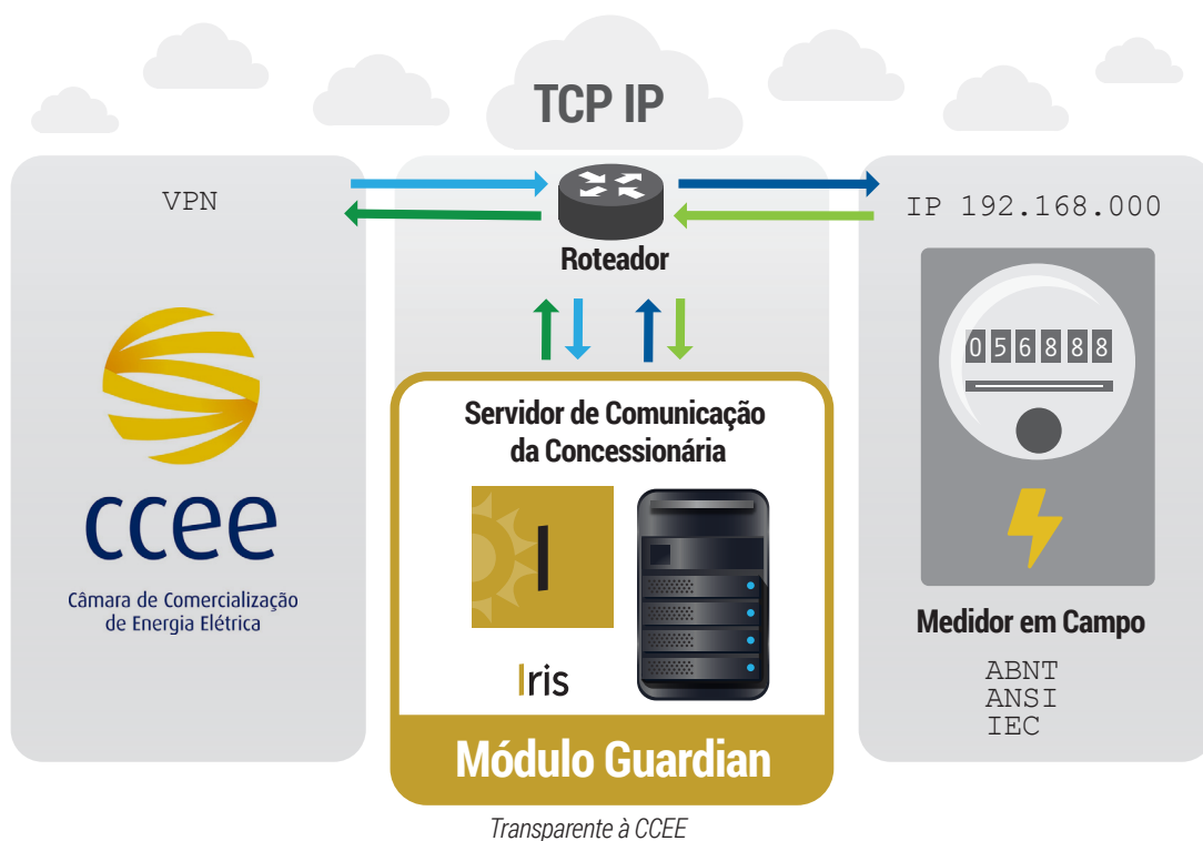
Ilustração do funcionamento do Módulo Port Forward
